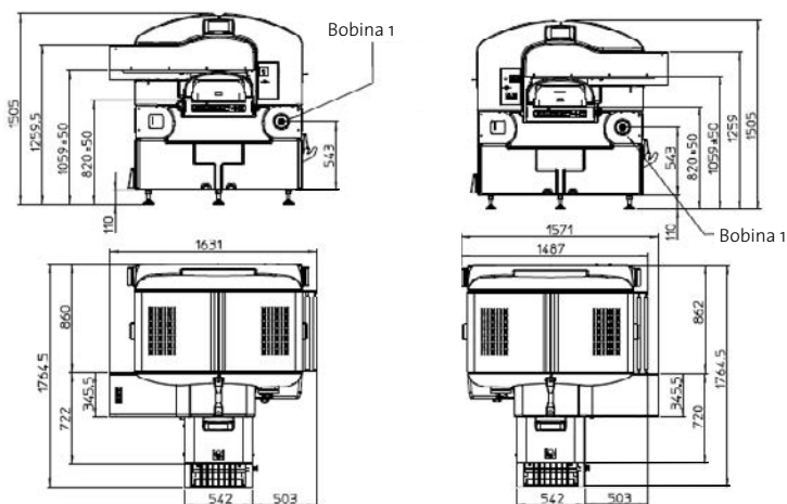
Automac 40 XL - Left
